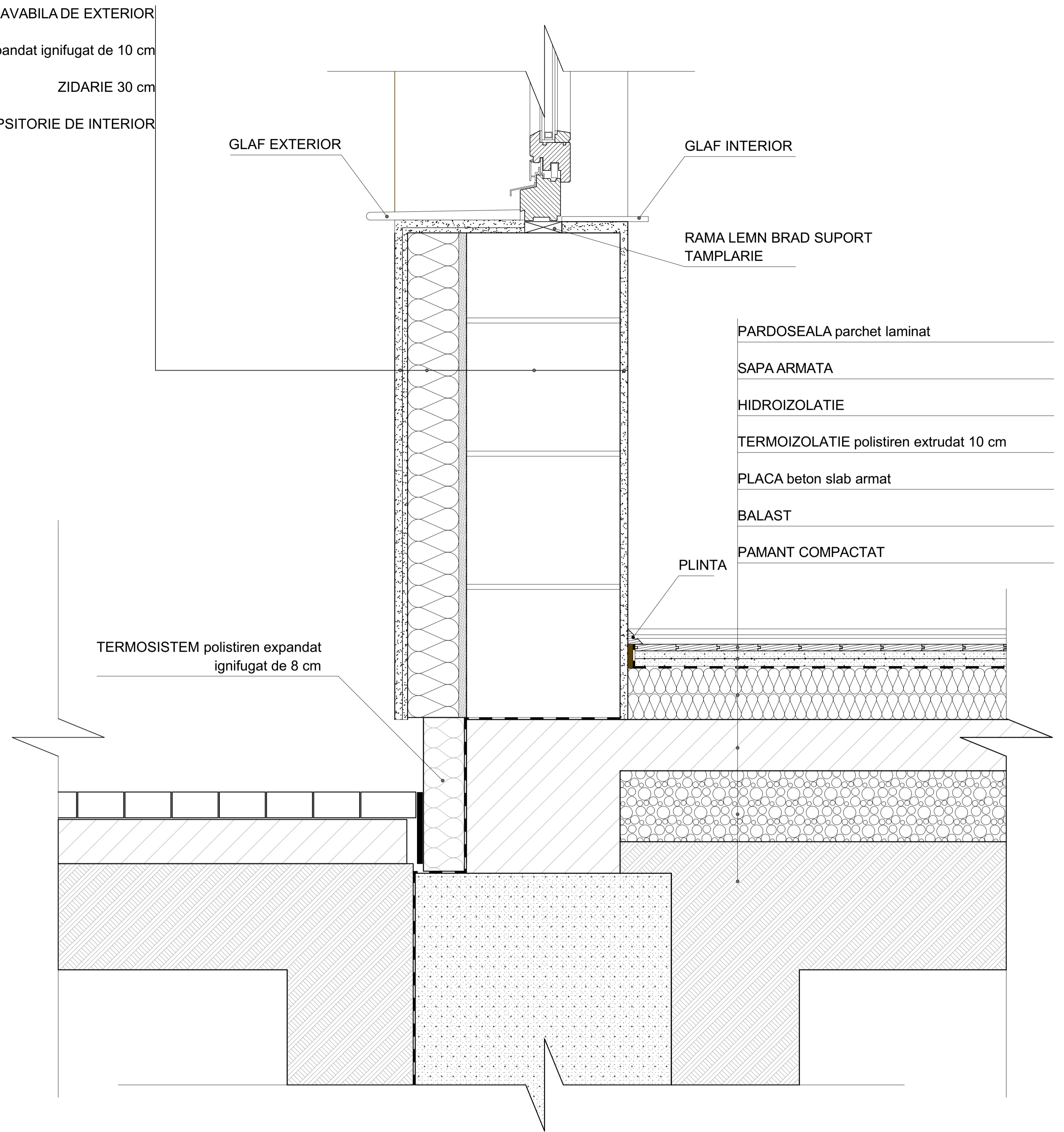
DETALIU 2 SCARA 1:5
