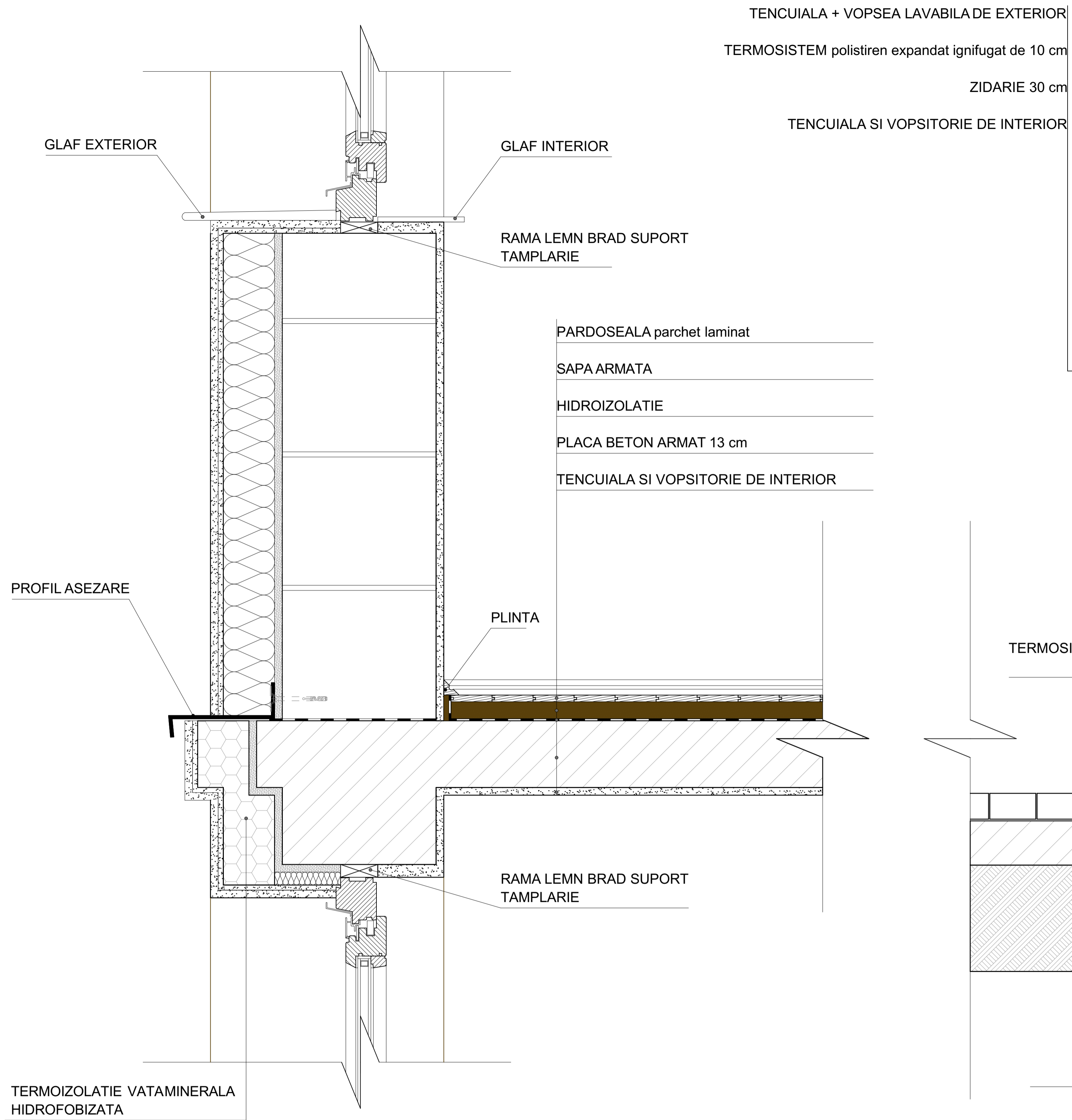
DETALIU 1 SCARA 1:5
