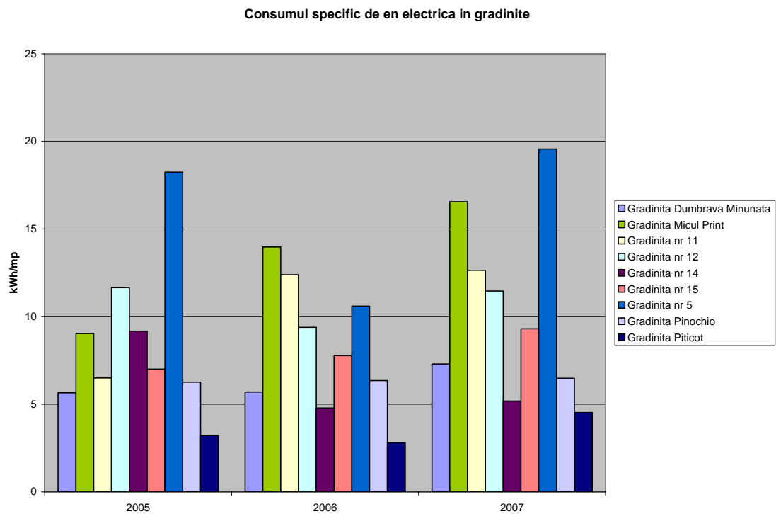
Fig.34. Consumul de energie electrica per mp suprafata utila in gradinitele din Medias
