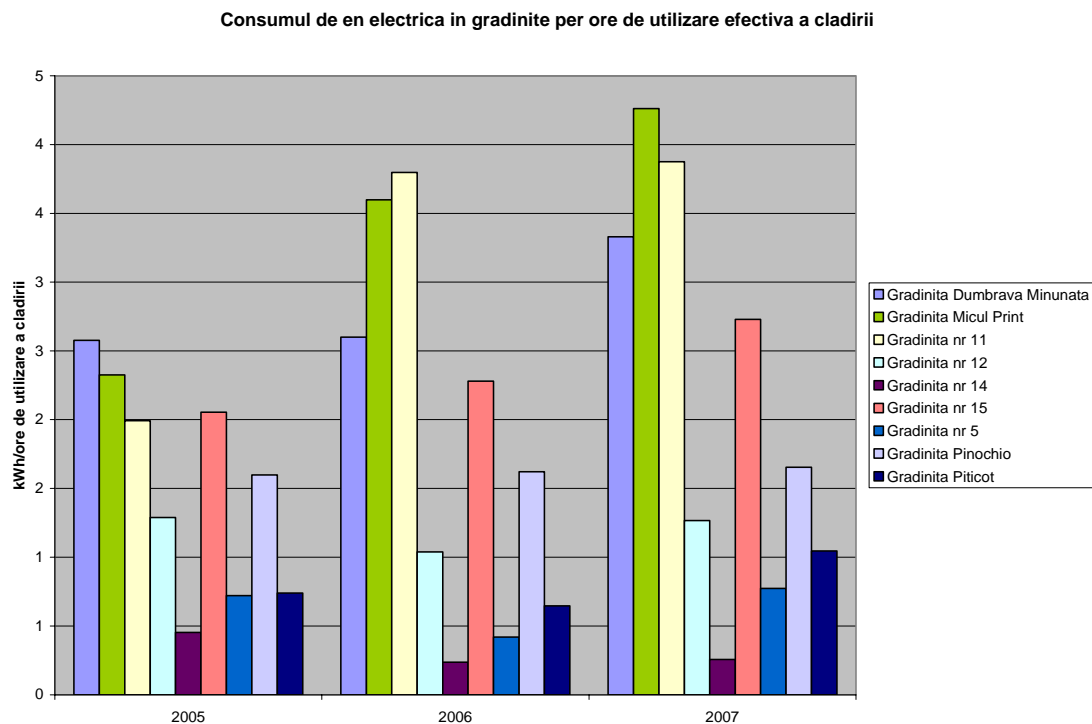
Fig.35. Consumul de energie electrica per ore de utilizare efectiva in gradinitile din Medias
