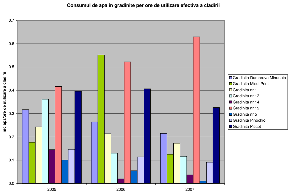
Fig.9. Consumul specific de apa per ore de utilizare efectiva a cladirii in gradinitele din Medias
