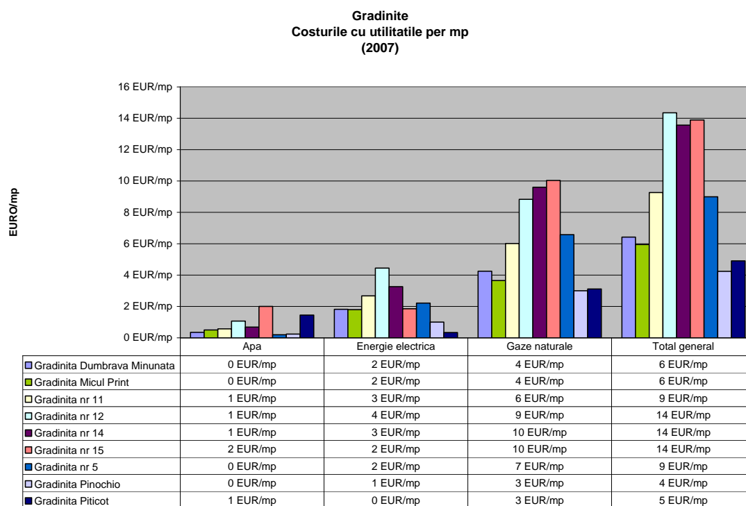
Fig.43. Costurile cu utilitatile per mp suprafata utila in anul 2007 in gradinitile din Medias
