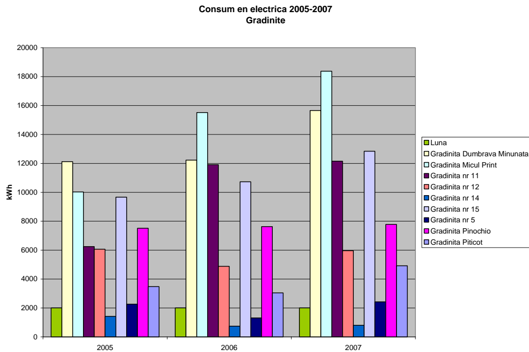
Fig.27. Consum cu energie electrica in gradinitile din Medias, in perioada 2005-2007
