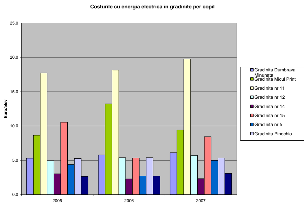
Fig.37. Costurile medii cu energia electrica per copil in gradinitele din Medias
