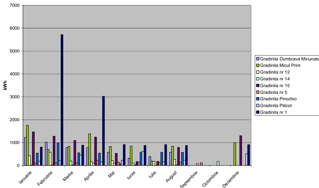
Fig.30. Consum cu energie electrica in gradinitile din Medias, in anul 2007
