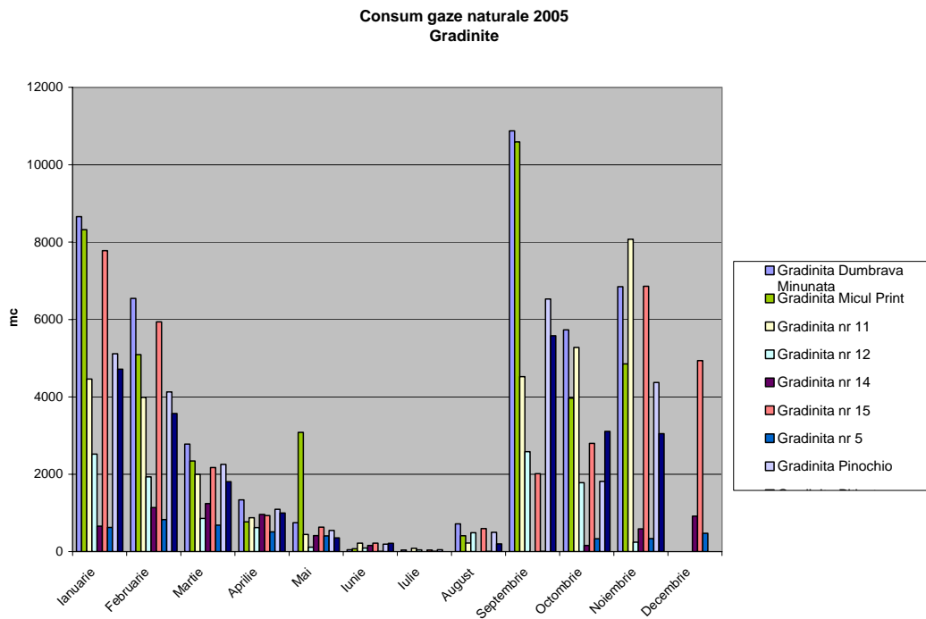
Fig.15. Consumul de gaze naturale in gradinitile din Medias, in anul 2005
