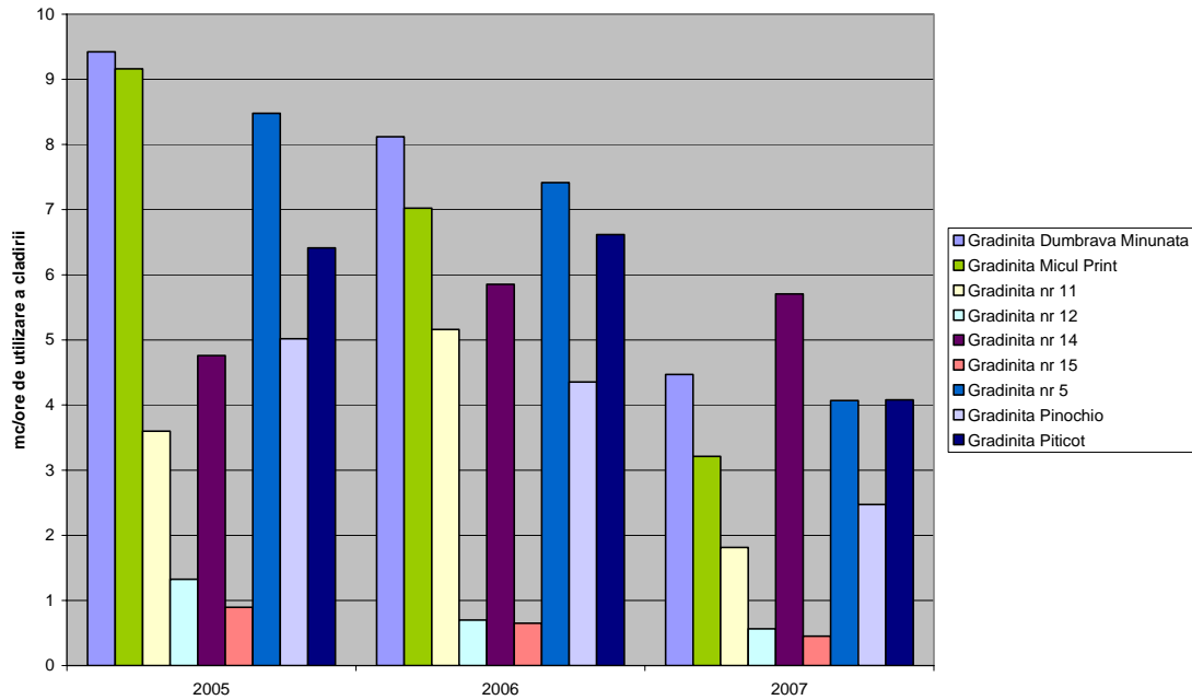
Fig.22. Consumul de gaze naturale per ore de utilizare efectiva a cladirii in gradinitile din Medias
