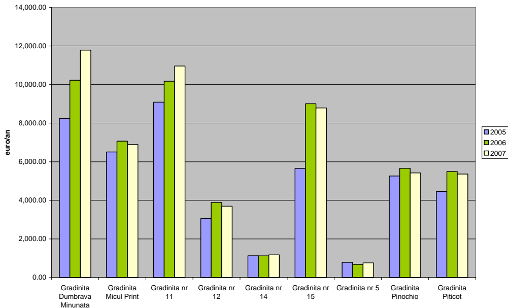
Fig.23. Costurile medii cu gazele naturale in gradinitile din Medias
