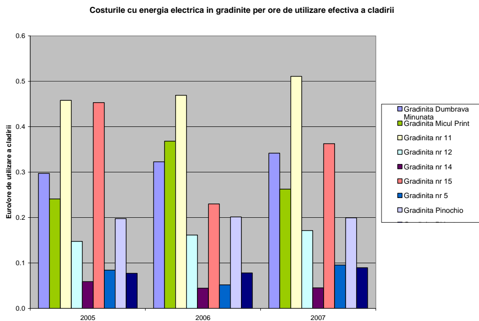
Fig.39. Costurile medii cu energia electrica per ore de utilizare efectiva a cladirii in gradinitele din Medias
