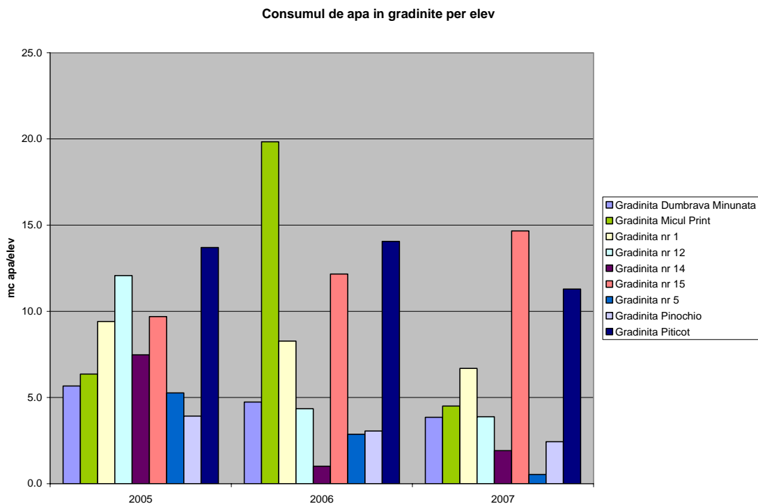
Fig.7. Consumul specific de apa per copil in gradinitele din Medias
