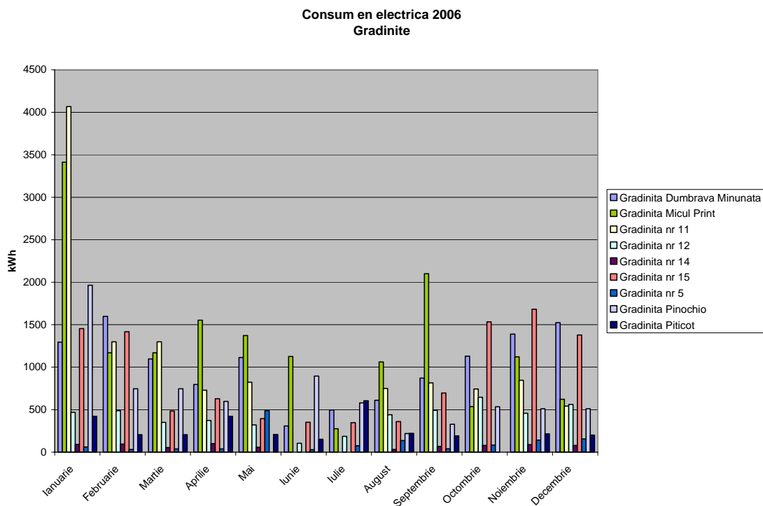
Fig.29. Consum cu energie electrica in gradinitele din Medias, in anul 2006
